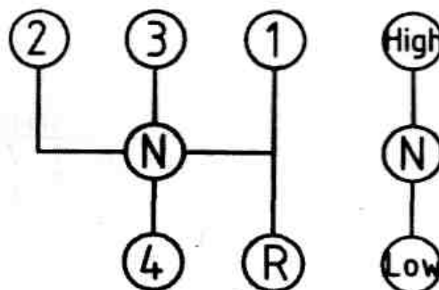
Рис.2.Схема переключения передач КПП.
